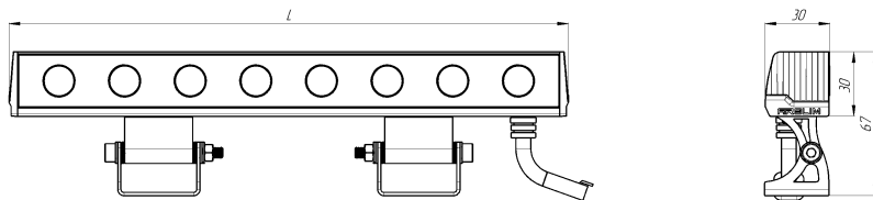
Рис.1. Габаритные размеры
